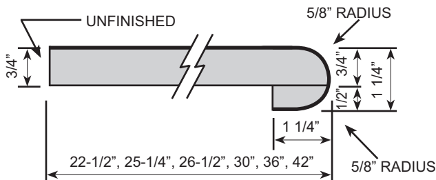
FLAT DECK TOP ETFV-22 1/2 ETFK-25 1/4 ETFB-26 1/2 ETFB-30 ETFB-36 ETFB-42
