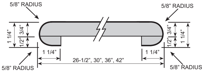
BAR TOP ETB-26 1/2 ETB-30 ETB-36 ETB-42
